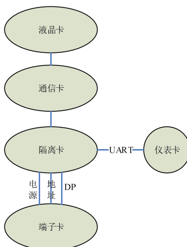
图 3.2 产品结构示意图
