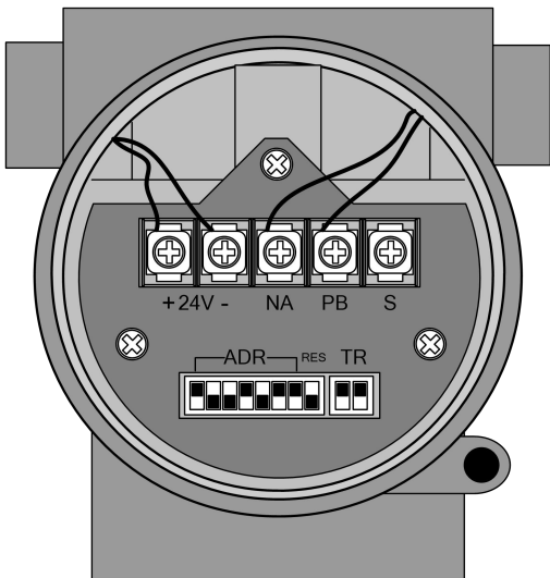
图 2.11 HART 型智能变送器接线图
