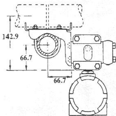
2.2 弯支架管装图
