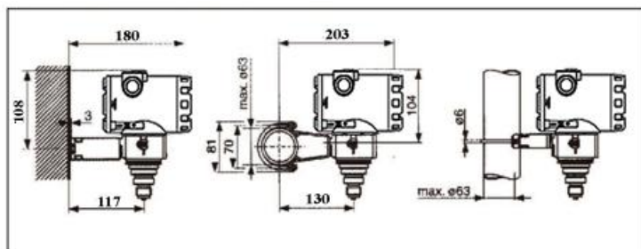
图 2.7 压力变送器安装方式
