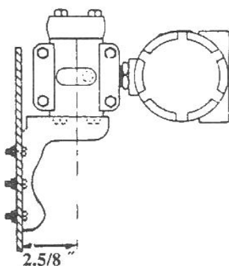
图 2.1 弯支架盘装图
