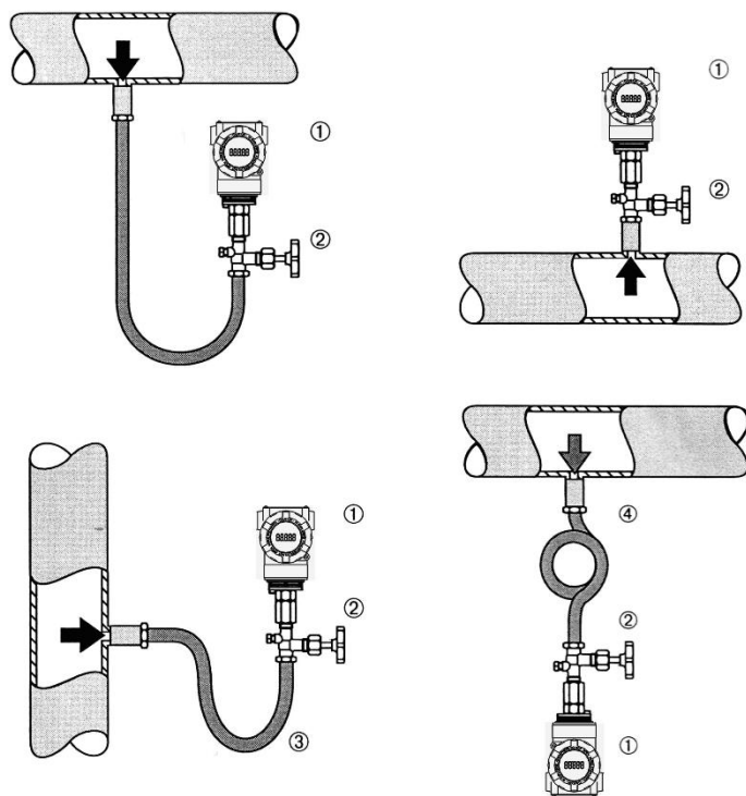
图 2.8 引压管连接示意图
