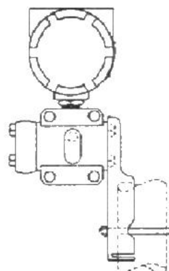
2.3 平支架管装
