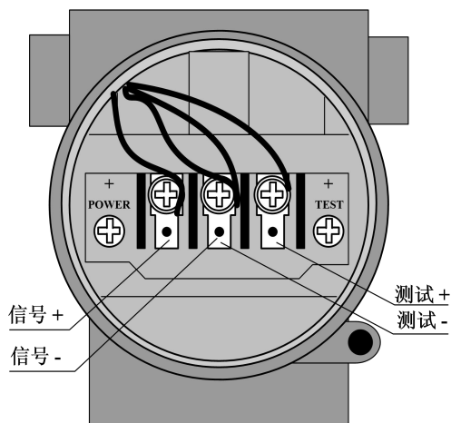
图 2.10 HART 型智能变送器接线图
