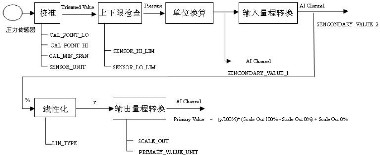
图 7.3 变换块结构
