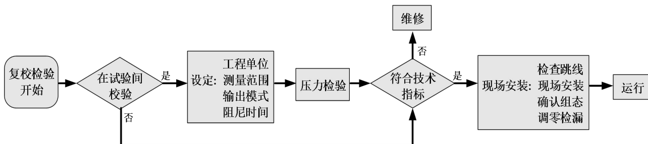
图 2.13 智能变送器复校检验流程
