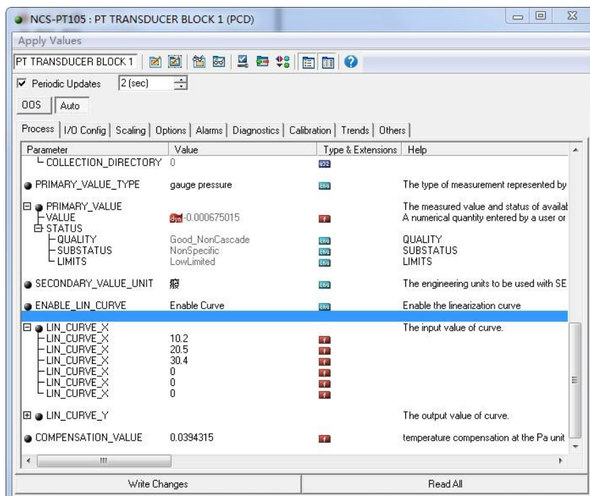
图 6.5 参数 LIN_CURVE_X 的配置
