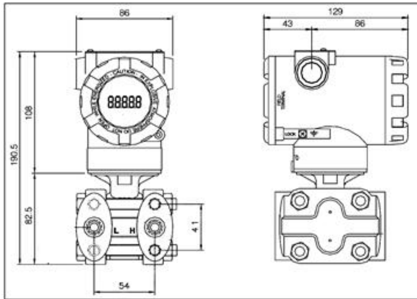
图 1.1 智能变送器外型尺寸（单位：mm）
