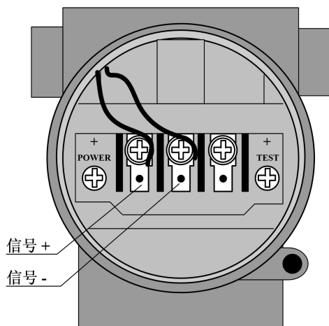
图 2.9 FF、PA 型智能变送器接线图
