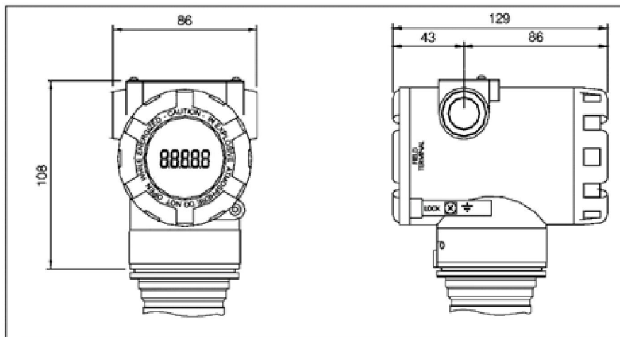
图 1.2 智能变送器外型尺寸（单位：mm）
