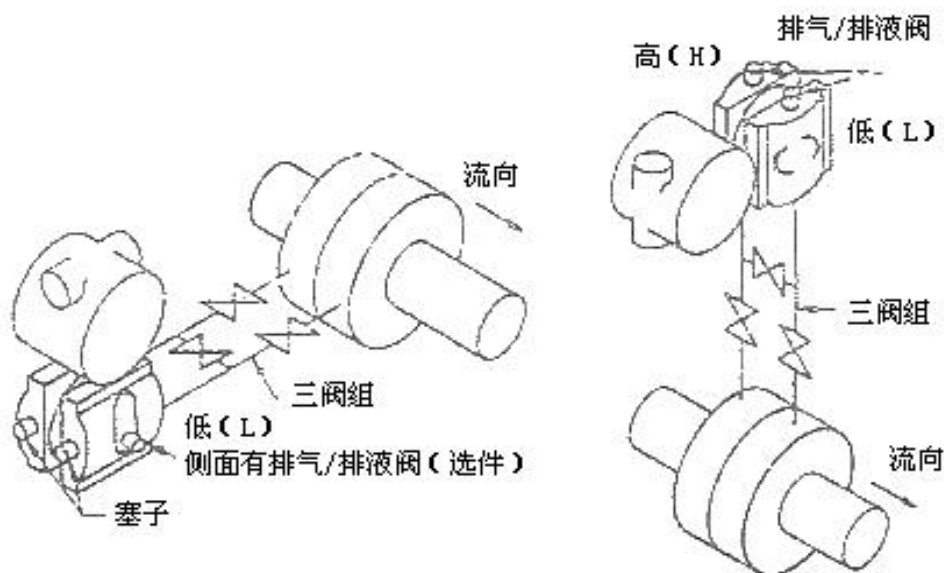
图 2.6 气体介质连接示意图
