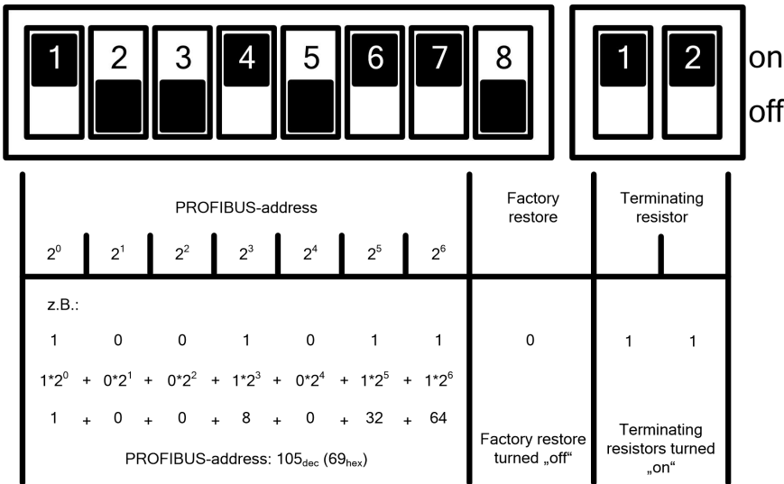
图 2.12 DIP 开关配置
